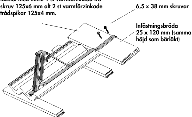
Bild 1. Montering av konsoll sker i takpannans dal.
