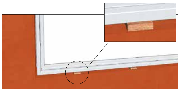
2. Sätt i och kila fast fönster/dörrkarm i lod.
