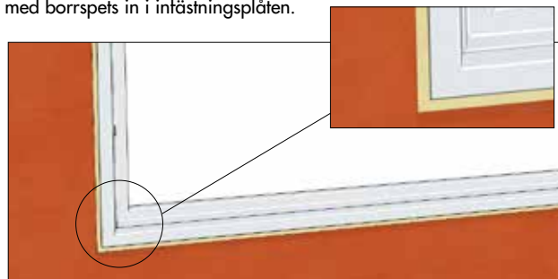
4. Dreva utrymmet mellan karm och murverk med isolering.
