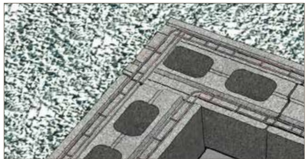
Bild 3.1 Armering av hörn
