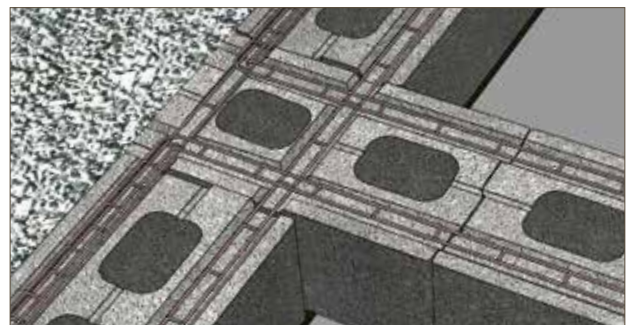
Bild 3.2 Armering av stödvägg
