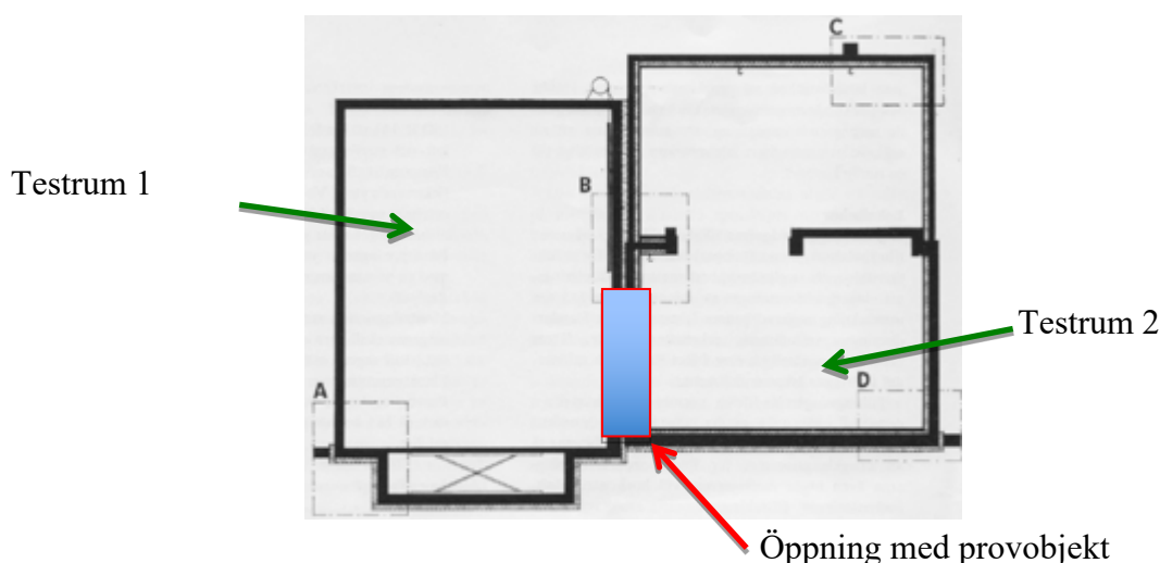
Figur B1.1: Sektion av laboratoriet med Testrum 2 (sändarrum) och Testrum 1 (mottagarrum, efterklangsrum). Provobjekten monteras i öppningen mellan rummen.
